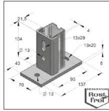
Wspornik 45 profilowy wzdłużny
