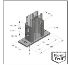
Wspornik profilowy szyny podwójnej 45/90
