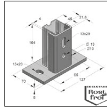
Wspornik 45 profilowy poprzeczny
