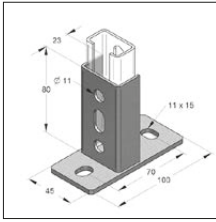
Wspornik 35 wzdłużny
